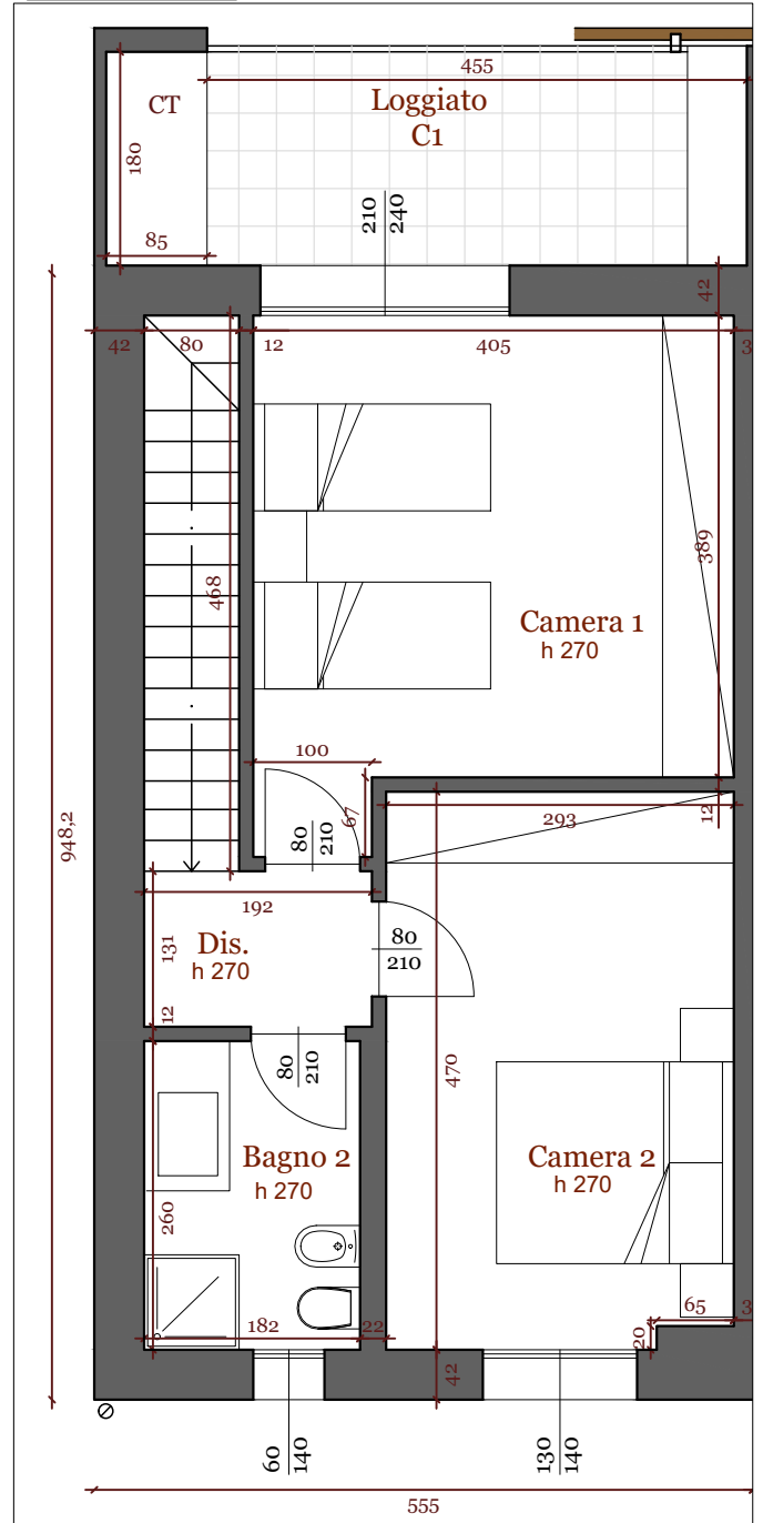
PIANO SECONDO
