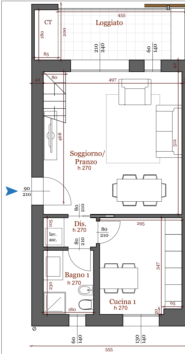
PIANO PRIMO
